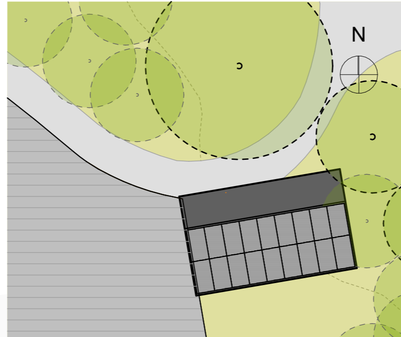
3. SITE PLAN 1:200
